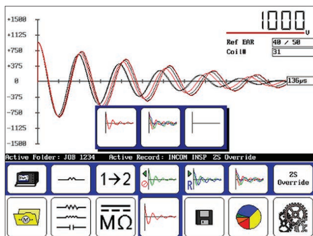
Импульсное испытание нескольких катушек
