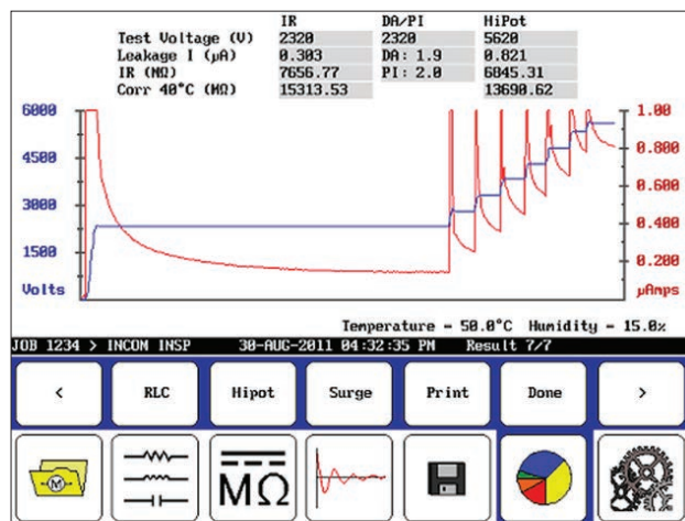
Результаты испытаний при постоянном токе
