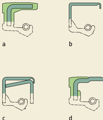
Конструкция наружного диаметра
