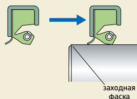
д) Монтаж по направлению кромки из PTFE
