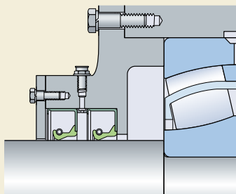
Парная установка уплотнений CRW1
