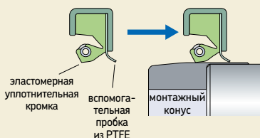
с) Монтаж против направления кромки из PTFE
