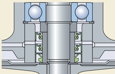
Уплотнения CRW5 + V-образное уплотнение
