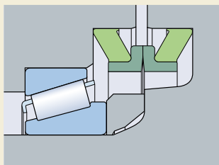
Механическое уплотнение HDDF с металлической парой трения
