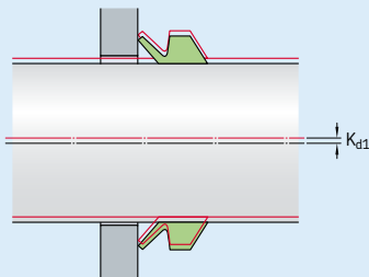
Допуски на соосность и радиальное биение валов
