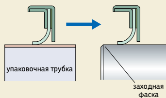
б) Монтаж по направлению кромки из PTFE
