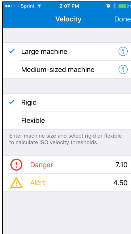
Рисунок 4 – 3. Таблица «Виброскорость».
